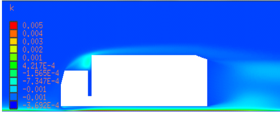
Fig. 17 Boat tail이 부착된 형상 난류 운동에너지 contour
