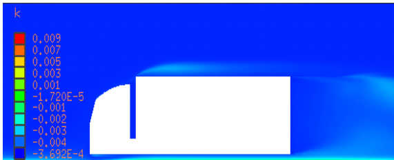
Fig. 18 Cap-roof fairing이 부착된 형상 난류 운동에너지 contour
